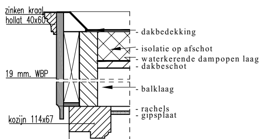
DETAIL 1 schaal 1:10
