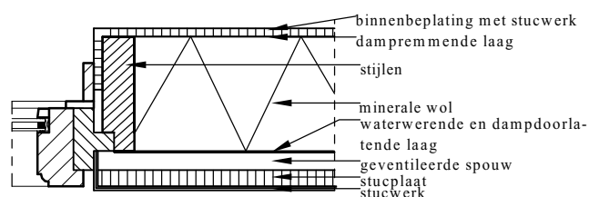
DETAIL 2 schaal 1:10
